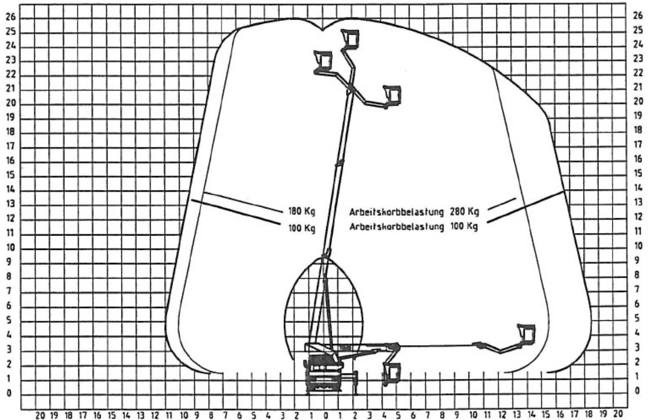
Kennfeld TKA 26 KS einseitige Abstützung Fahrzeugbedingte Änderungen vorbehalten
